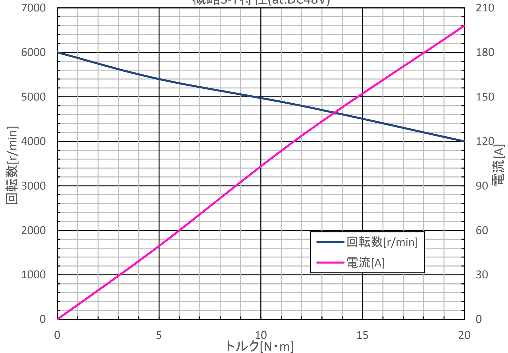
概略S-T特性(at.DC48V)
